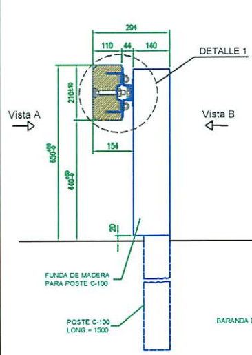
SECCIÓN RECTA A-A' Escala: 1/10
