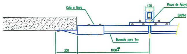
Planta
