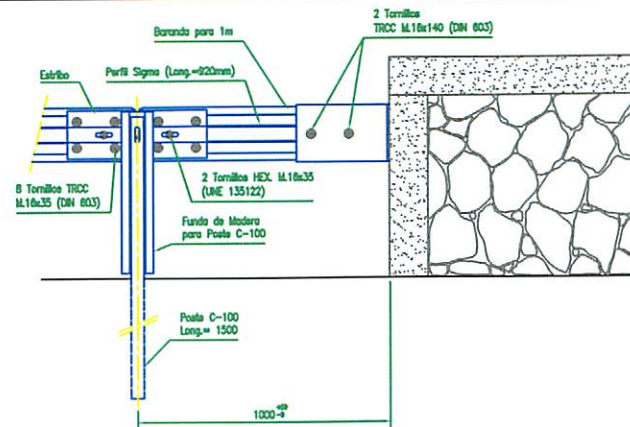
Alzado Posterior
