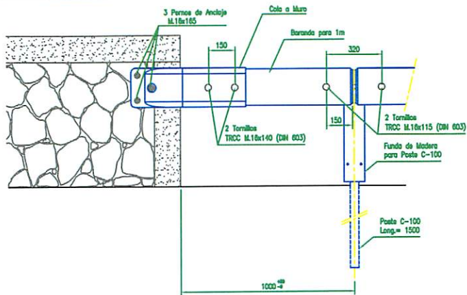
Alzado
